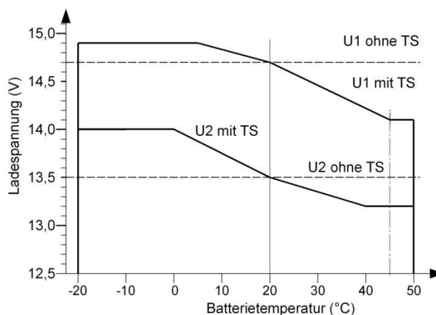
Ladeprogramm „AGM / Vlies“, Kennlinie IU1oU2
