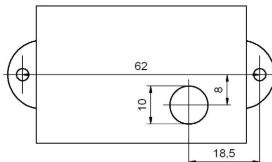
Geräteoberkante
