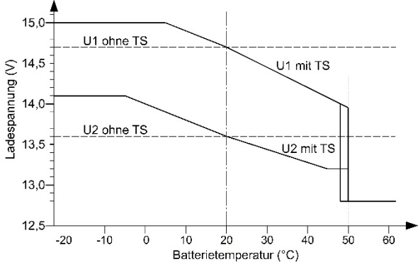
Ladeprogramm „AGM2“, Kennlinie IU1oU2
